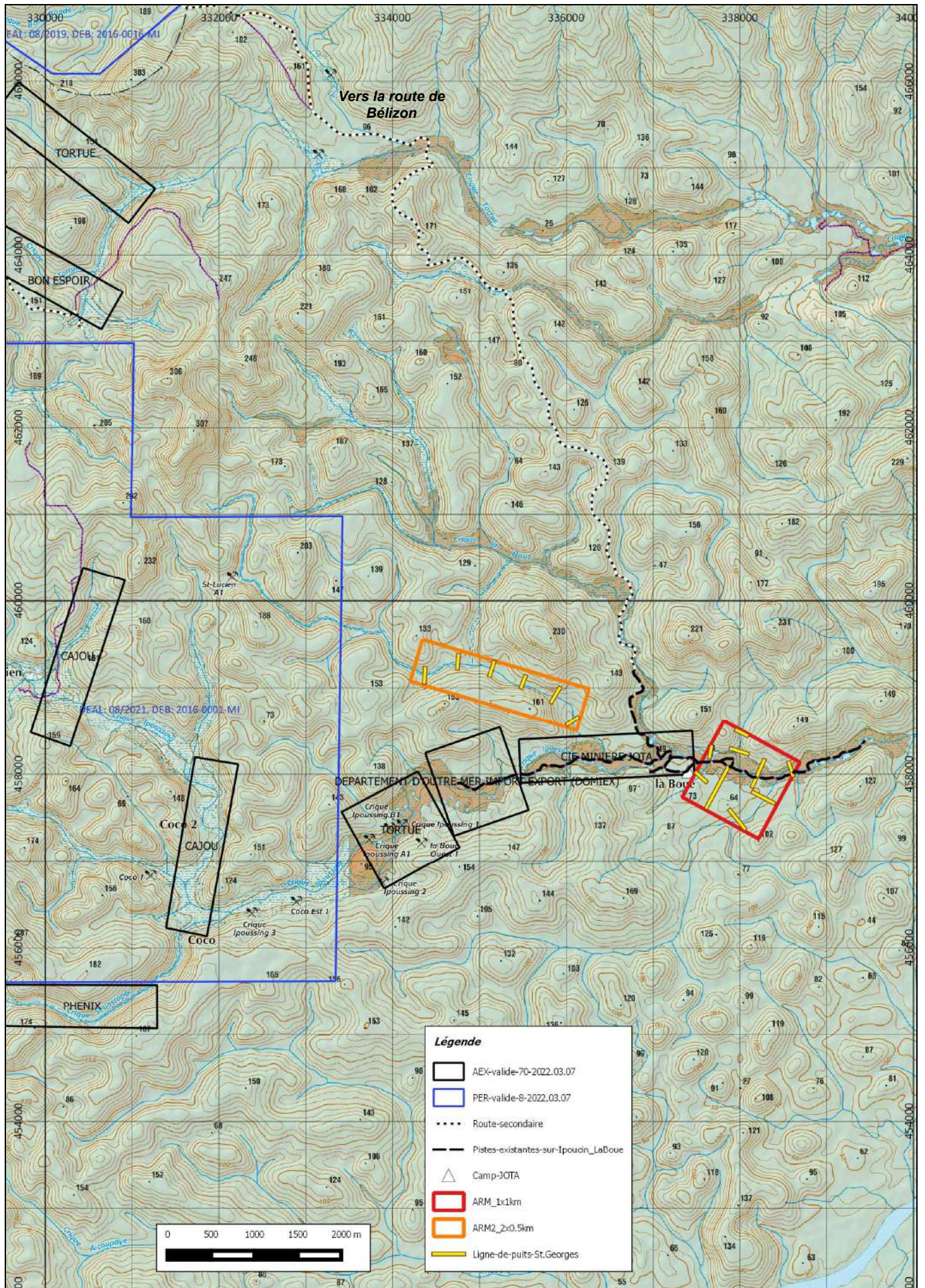
Annexe 4a : Schéma de pénétration du domaine forestier / ARM de l'EURL SAINT-GEORGES d'après la carte IGN au 1/50 000 e en RGFG95, UTM22
