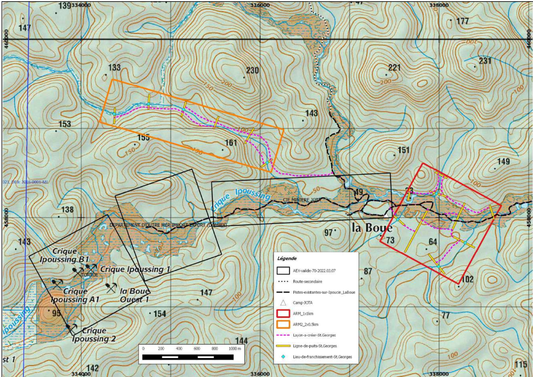
Annexe 4b : Plan de projet dans le cadre de l'ARM « criques Ipooussing-Est et Calou » de l'EURL SAINT-GEORGES d'après la carte IGN au 1/20 000° en RGFG95, UTM22
